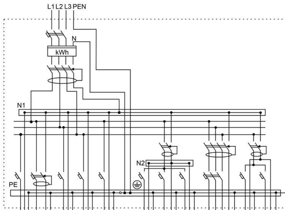
Рисунок 6. Схема квартирного учетно-группового щитка (для коттеджа)*
