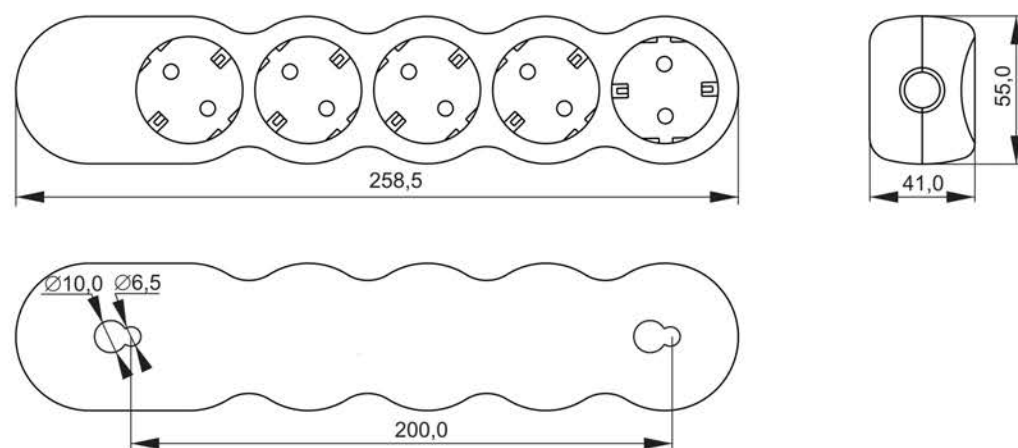
Рисунок 2 – Колодка удлинителя Y05
