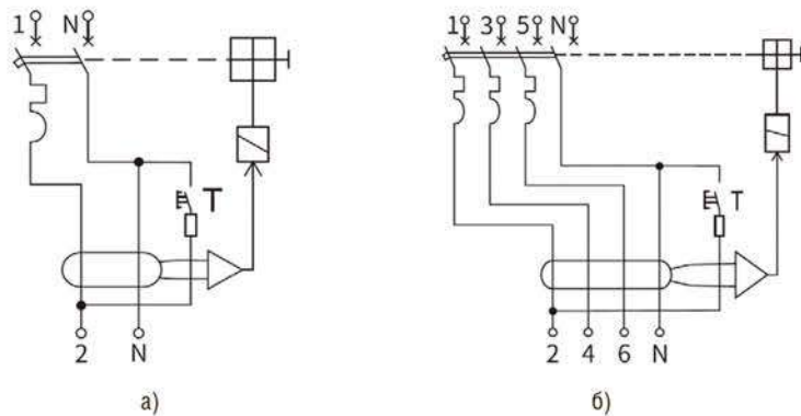
Рисунок Г.1 а) двухполюсного; б) четырехполюсного Т – устройство эксплуатационного контроля (кнопка «ТЕСТ») R – токоограничивающее сопротивление
