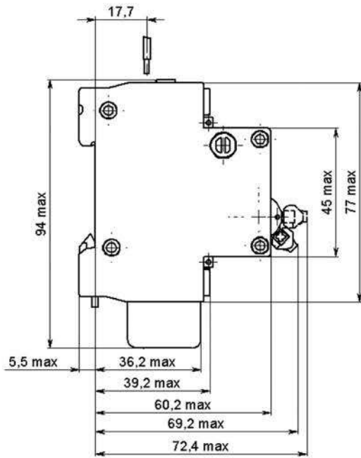
б) Рисунок В.1 а) АД12; б) АД14
