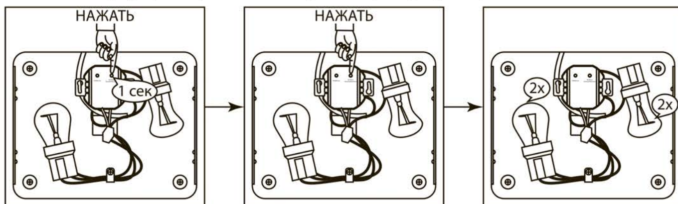
Рисунок 9. Удаление всех кодов из приемника M1
