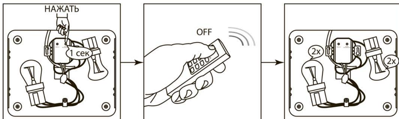
Рисунок 8. Пример отключения пультов ПУЗ, ПУБ от приемника M1
