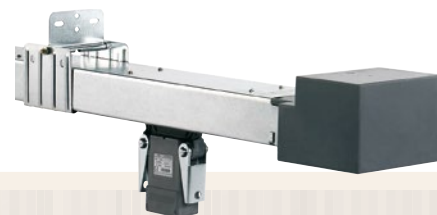
ТРОЛЛЕЙНЫЕ ШИНОПРОВОДЫ СЕРИИ TS ОТ 63 А ДО 250 А ТРЕХФАЗНЫЕ (3L+N+PE)
