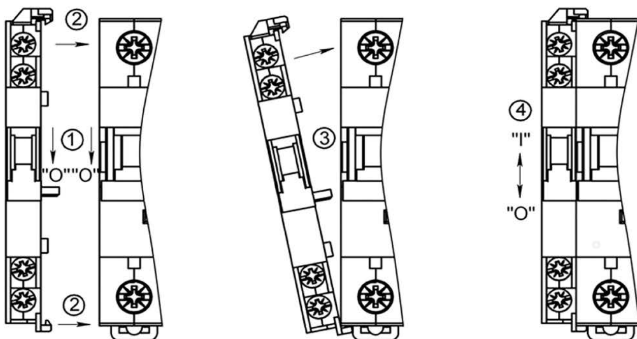
Рисунок Д.1 - Присоединение OptiDin MCK1, OptiDin MCK2, OptiDin MССК2 к выключателю
