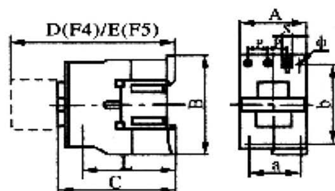
Рисунок 1- Габаритные и установочные размеры контактора NC1-09-32
