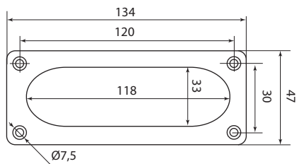
Фланец для установки KBM-10
