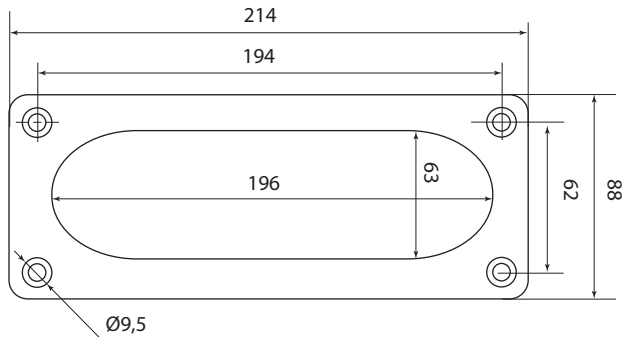
Фланец для установки KBM-6/16/25/35/50
