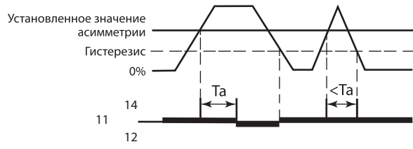
Схема работы реле PH (кроме моделей PH 04, PH 05, PH 12) при асимметрии фаз.
