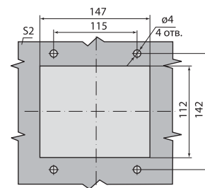
Шаблон для разметки и сверления металлической панели
