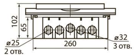
ЩРВ-П-24
