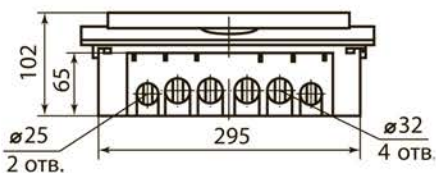
ЩРВ-П-36
