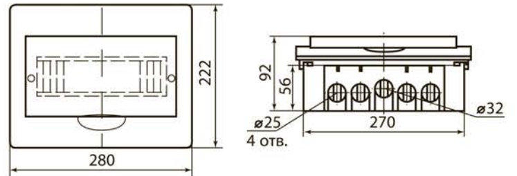
ЩРВ-П-12
