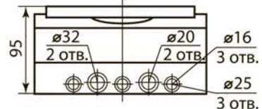
ЩРН-П-6
