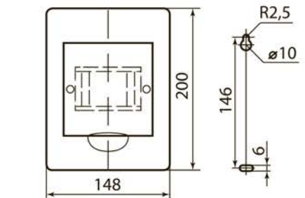
ЩРН-П-6
