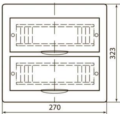
ЩРН-П-15
