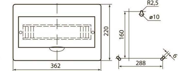
ЩРН-П-18
