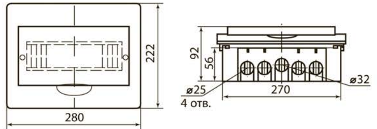
ЩРВ-П-12
