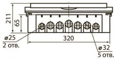
ЩРВ-П-15
