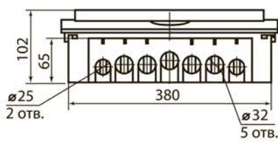
ЩРВ-П-18
