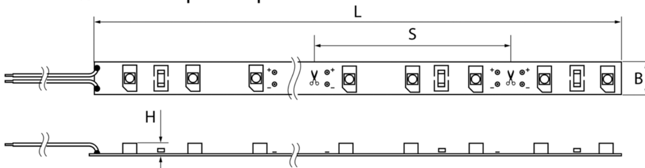
Рис. 1 Лента светодиодная
