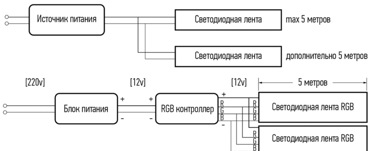
Рис. 2 Подключение светодиодной ленты
