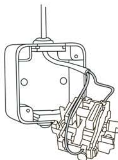
3.5. Прикрепить корпус изделия к стене двумя шурупами (в комплект не входят). Продеть кабель в отверстие в сальнике. Зачищенные провода, нажав на зажимы клеммы, вставить в контакты. Отпустить зажимы клемм.
