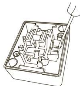
3.3. Снять механизм с направляющих.
