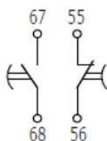
Рисунок Б.10 - Приставки выдержки времени типов: ПВЛ-11, ПВЛ-12, ПВЛ-13
