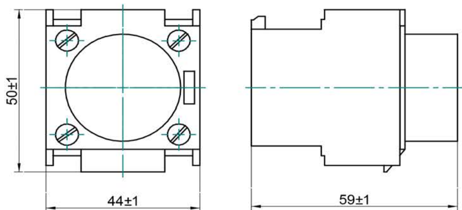
Рисунок А.6 Приставки выдержки времени типов: ПВЛ-11, ПВЛ-12, ПВЛ-13, ПВЛ-21, ПВЛ-22, ПВЛ-23
