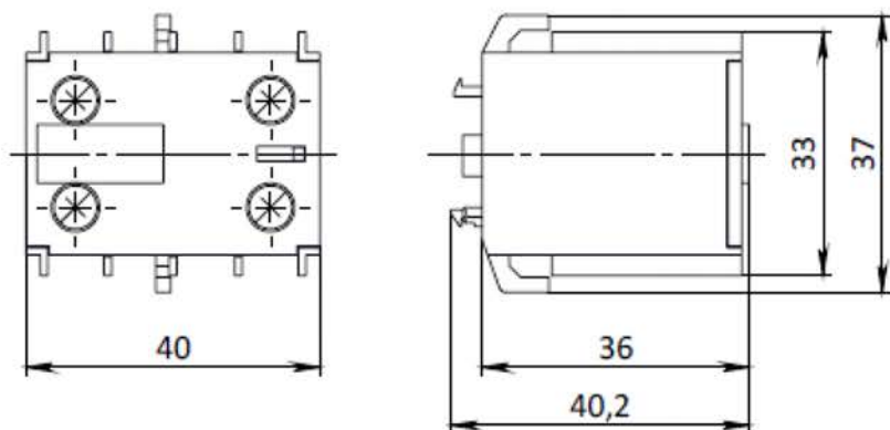
Рисунок А.3 – Приставки контактные типов: ПКЛ-М02, ПКЛ-М20, ПКЛ-М11
