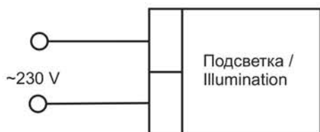
Рисунок 1 – Схема подключения
