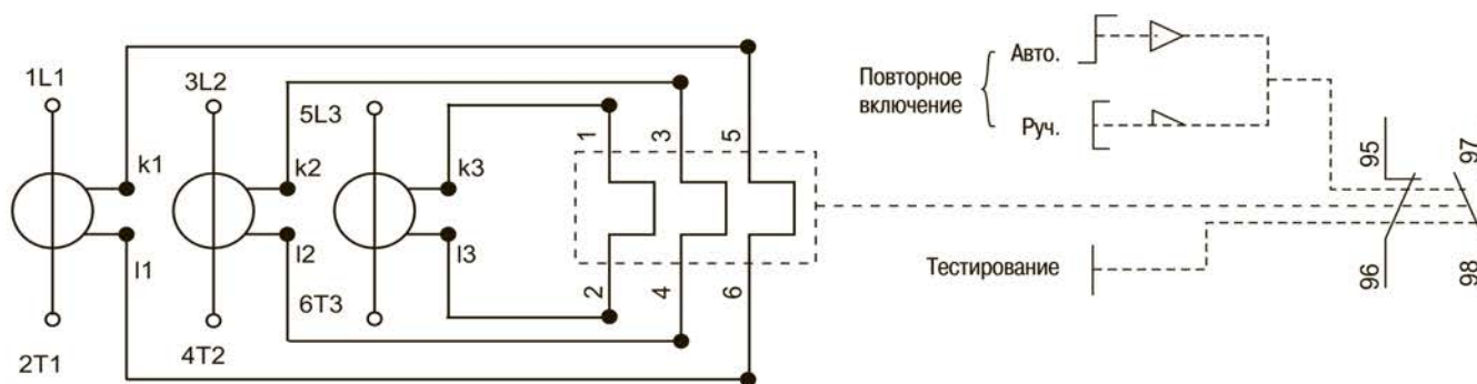
Рис. 3 Схема реле РТЭ-53125
