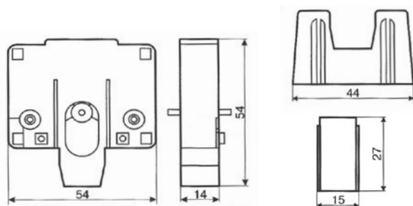
Блокировочное устройство до 32 А
