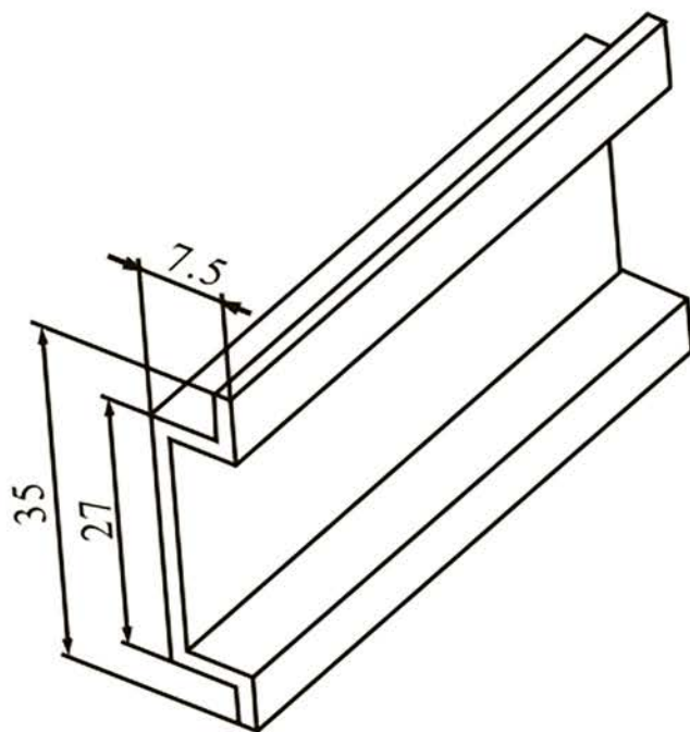
TH35-7.5 DIN rail
