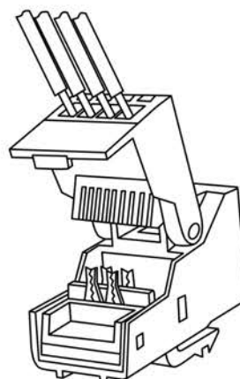
Рисунок 4. Расположить провода в джеке согласно разметке.
