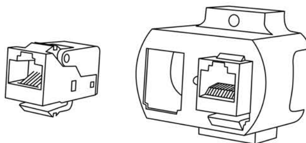
Рисунок 2. Извлечь джек из пластикового суппорта.
