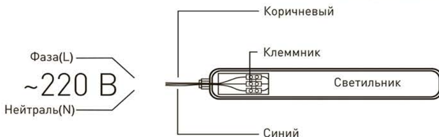
Рис.1. Схема подключения светильника к сети 220В.
