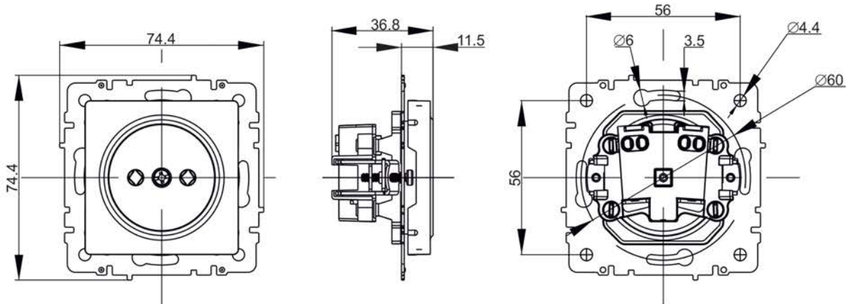
б) PC10-1-0-БрХ*; РСш10-2-БрХ*
