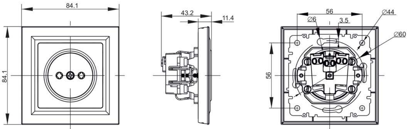
а) PCP10-1-0-БрХ*
