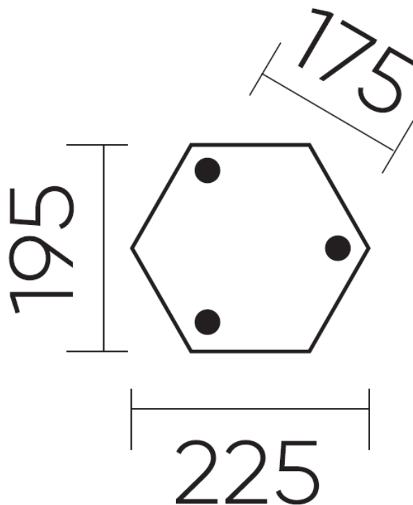
Схема основания светильника
