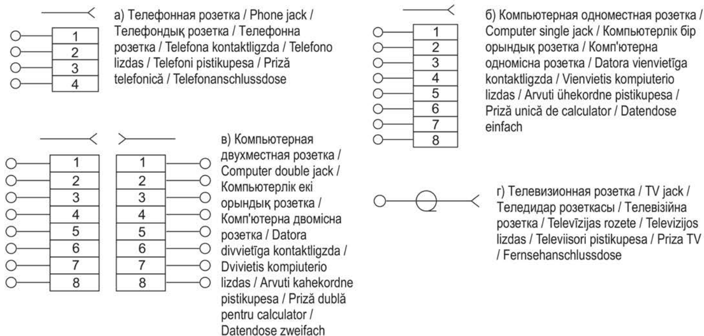
Рисунок 1 – Электрические схемы телефонных розеток / Figure 1 – Electrical schematics of phone jacks / 1-сурет – Телефон розеткаларының электр схемалары / Рисунок 1 – Електричні схеми телефонних розеток / 1. attēls – Telefona kontaktligzdas elektroinstalācijas shēmas / Pav. 1 – Telefono lizdų elektros schemas / Joonis 1 – Telefoni pistikupesade ühendusskeemid / Figura 1 – Scheme de cablare pentru prizele telefonice / Bild 1 – Schaltpläne der Telefonanschlussdosen
