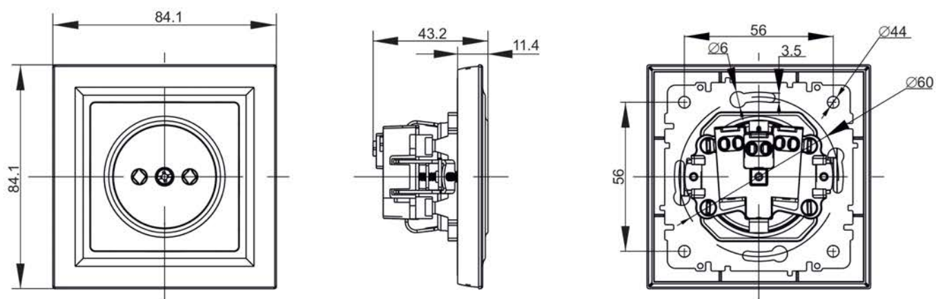
а) PCP10-1-0-БрХ*
