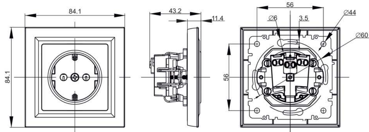
в) PCP14-1-0-БрХ*
