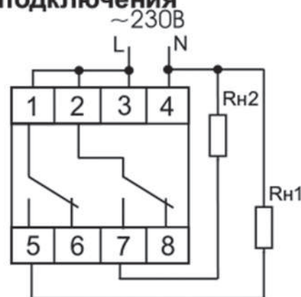
Рис.1 Рекомендуемая схема подключения таймера PCZ-527 и нагрузки к сети 230 В.
