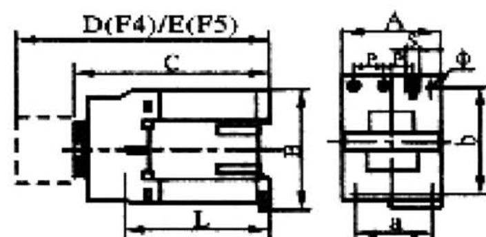
Рисунок 3- Габаритные и установочные размеры контактора NC1-09Z~32Z
