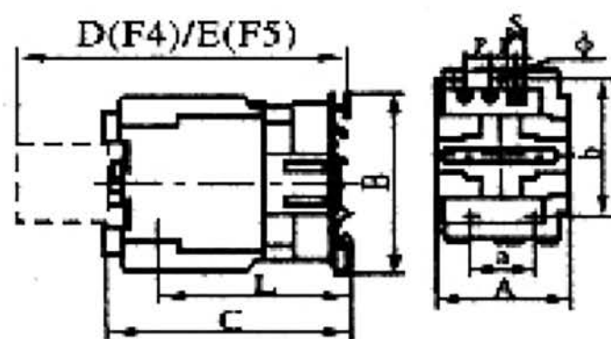
Рисунок 2- Габаритные и установочные размеры контактора NC1 40-95
