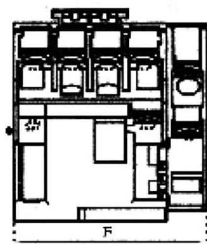
Рисунок 5- Габаритные и установочные размеры контактора NC1-09-32
