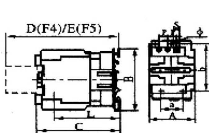
Рисунок 2- Габаритные и установочные размеры контактора NC1 40-95
