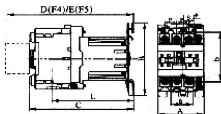
Рисунок 4- Габаритные и установочные размеры контактора NC1-40Z~95Z
