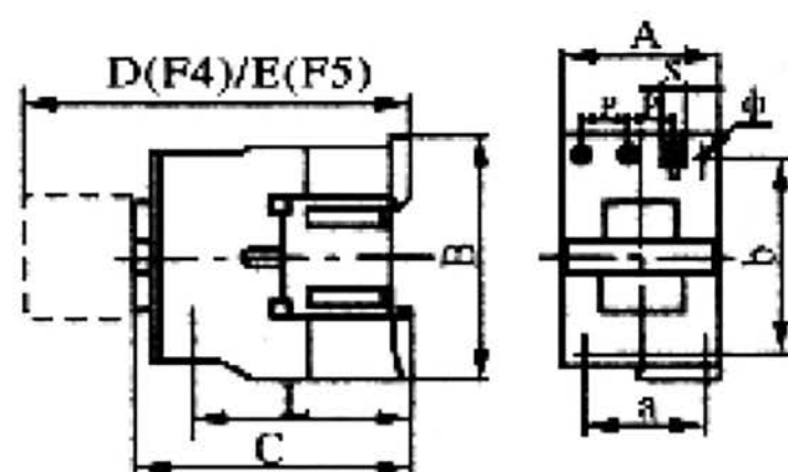
Рисунок 1- Габаритные и установочные размеры контактора NC1-09-32
