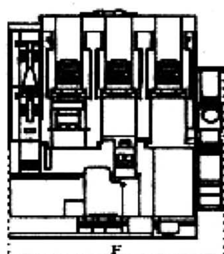
Рисунок 6- Габаритные и установочные размеры контактора NC1-40-95
