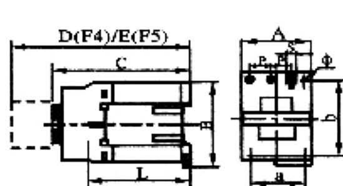
Рисунок 3- Габаритные и установочные размеры контактора NC1-09Z~32Z
