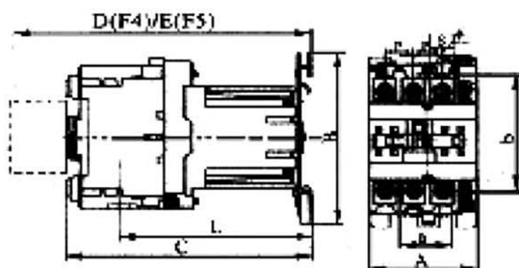
Рисунок 4- Габаритные и установочные размеры контактора NC1-40Z~95Z
