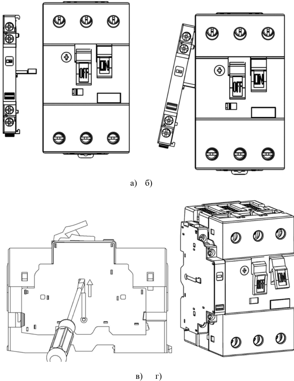
Рисунок 3. Способ сборки пускателя NS2-AU (80B)
