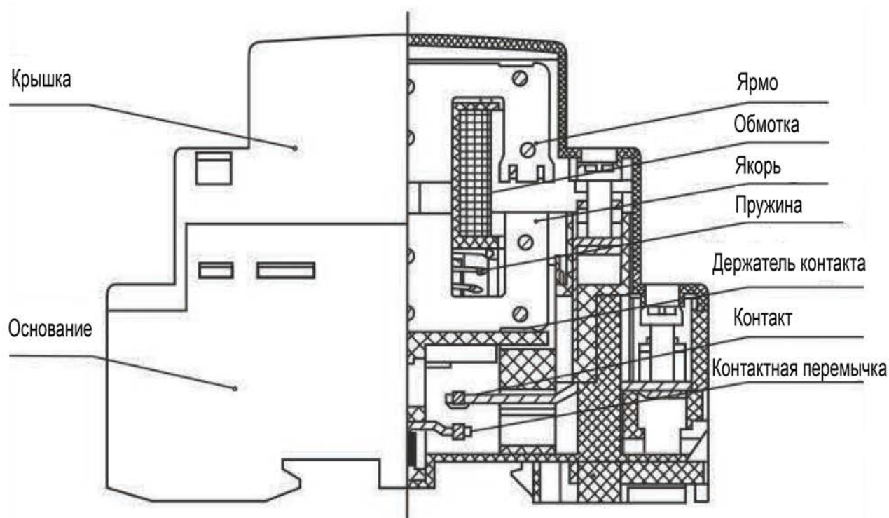
Рисунок 1. Основные элементы конструкции контактора
