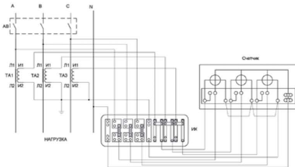
Рисунок 1 - Схема подключения коробок
