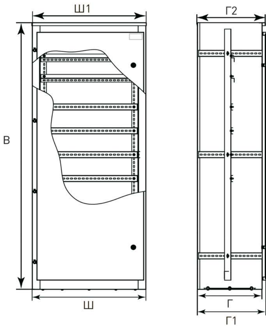
Рис. 1 - Общий вид шкафов ШРС IP54
