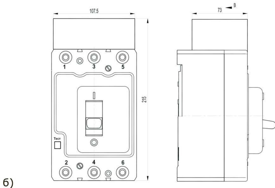
Рисунок Б.1 - Выключатель BA57-35 (BA57Φ35) с зажимами для переднего присоединения
