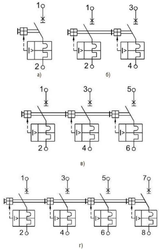
Рисунок Г.1 а) однополюсного; б) двухполюсного с двумя защищенными полюсами; в) трёхполюсного с тремя защищенными полюсами; г) четырёхполюсного с четырьмя защищенными полюсами.
