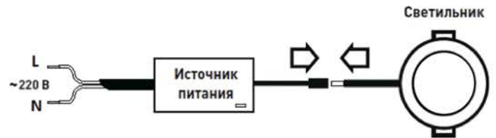
Рис.1. Подключение светильника к сети переменного тока 220В.
