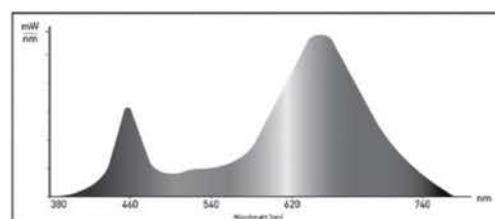
СПЕКТРОГРАММА ИЗЛУЧЕНИЯ
