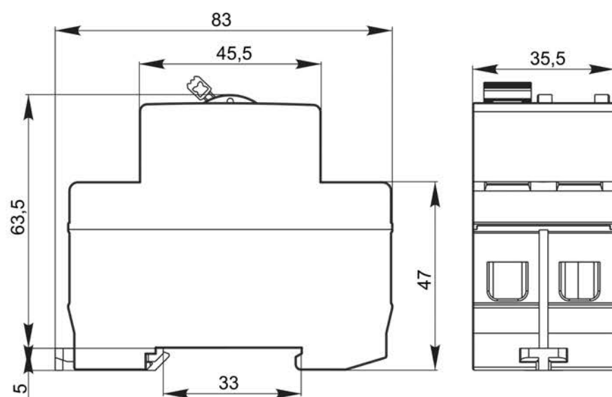
а) Двухполюсные ВД
