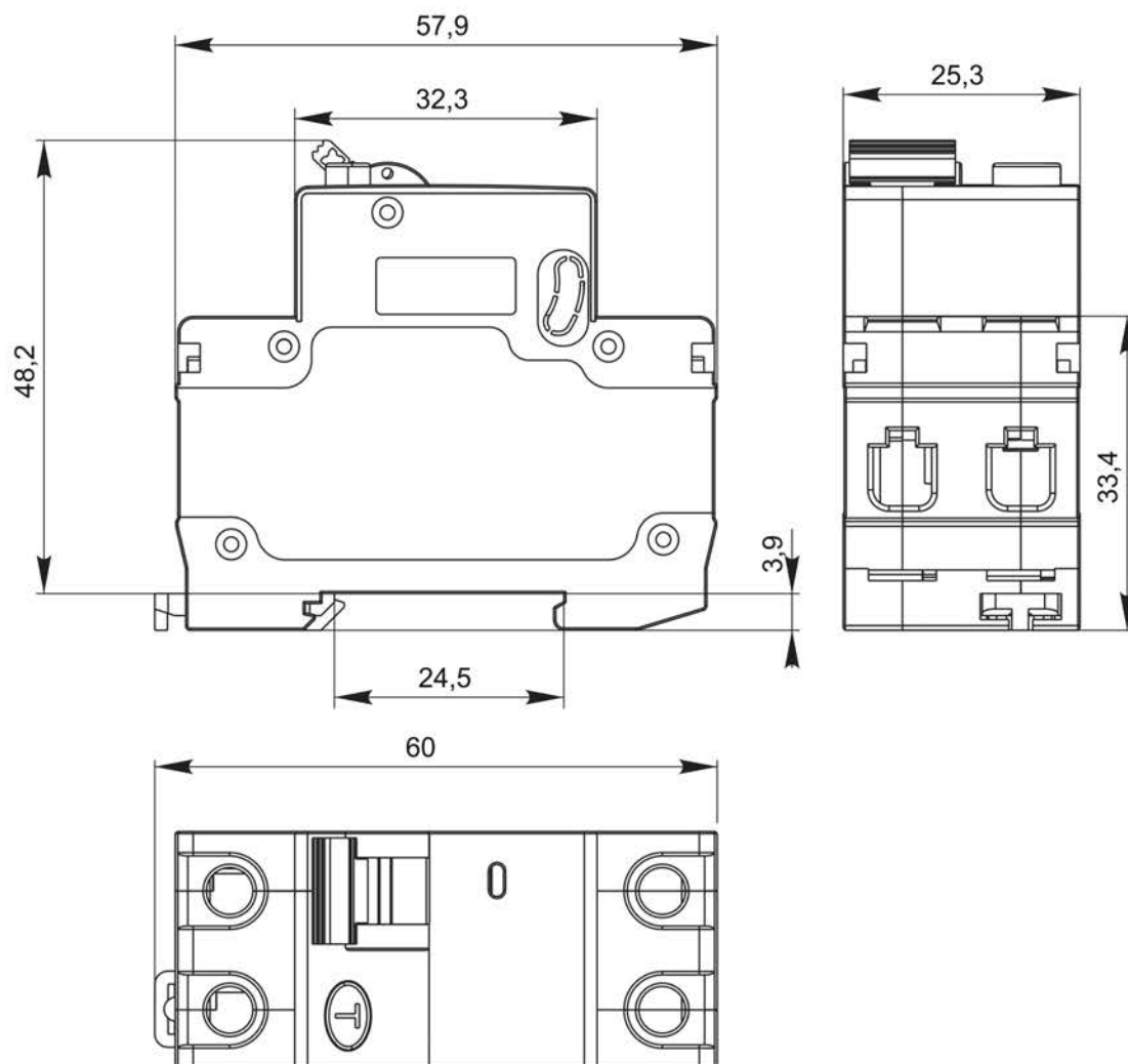
Рисунок 1 – Габаритные и установочные размеры АВДТ
