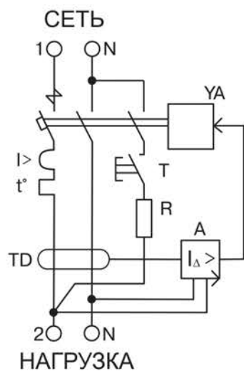
Рисунок 2 – Схема электрическая принципиальная
