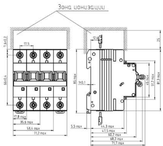
Рисунок В.1– Габаритные и установочные размеры выключателей
