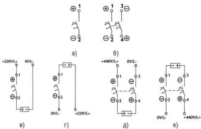
а) однополюсного; б) двухполюсного и примеры подключения в сетях постоянного тока в), г) однополюсного; д),е) двухполюсного Рисунок Г.2 – Принципиальные электрические схемы выключателей постоянного тока
