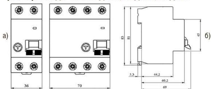
Рисунок В.1 – Габаритные, установочные и присоединительные размеры АВДТ
