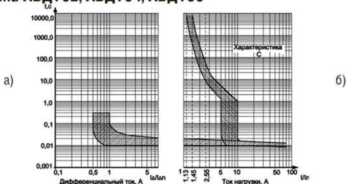
Рисунок Б.1 – Время-токовые характеристики отключения АВДТ
