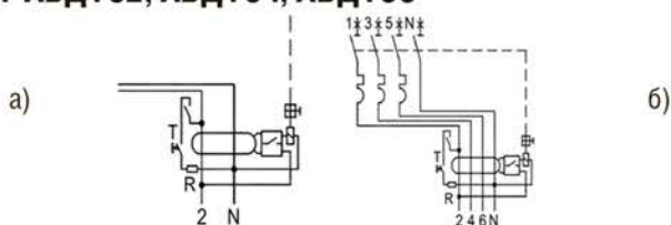
Рисунок Г.1 – Принципиальные электрические схемы АВДТ
