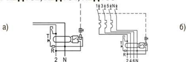
Рисунок Г.1 – Принципиальные электрические схемы АВДТ
