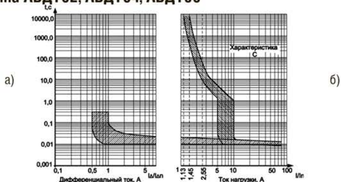
Рисунок Б.1 – Время-токовые характеристики отключения АВДТ
