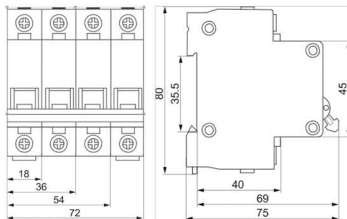
Рисунок Б.1 Габаритные, установочные, присоединительные размеры выключателей.
