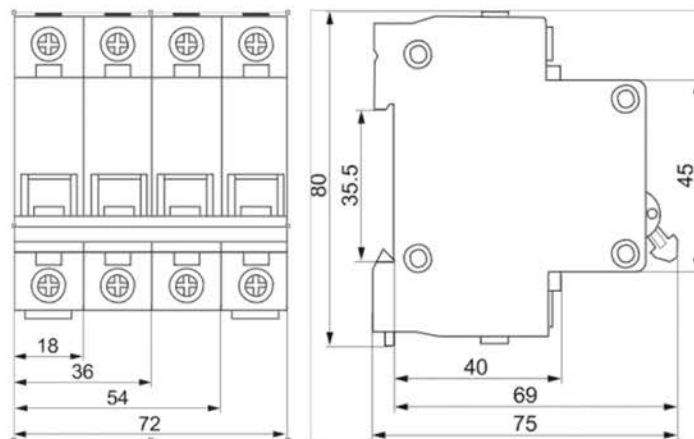
Рисунок Б.1 Габаритные, установочные, присоединительные размеры выключателей.
