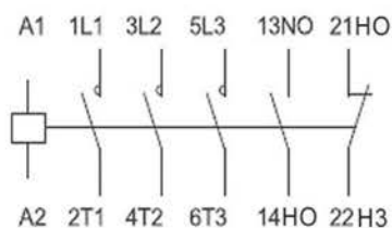
KM-103 9-95A
