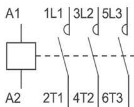
KM-103 115-630A
