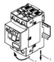
Рис. 3. Демонтаж автоматического выключателя ВА-431 с дин-рейки.
